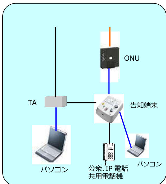
図 3. ISDN の接続構成
