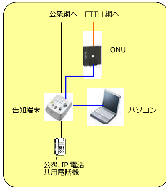
図 2. ADSL を解約した場合の接続構成
