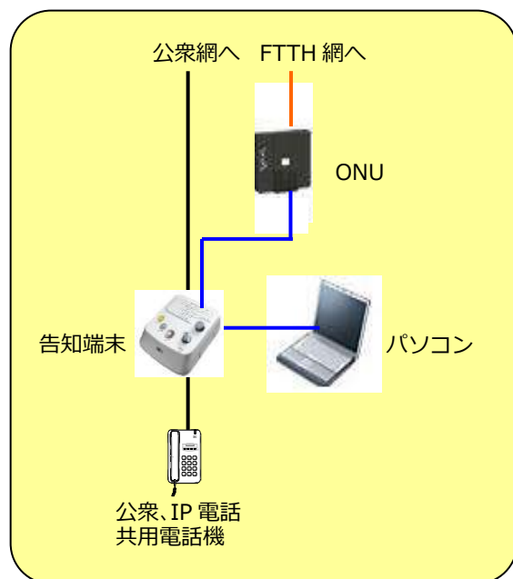
図 4. ISDN を解約した場合の接続構成
